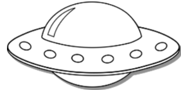
a UFO
